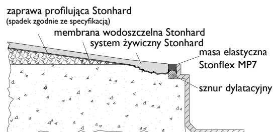
KANAŁ DRENAŻOWY Prefabrykowany kanał drenażowy z membraną
