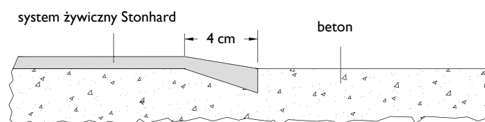
WCIĘCIE W POSADZCE
