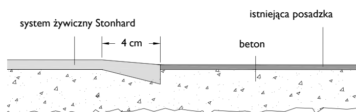
POŁĄCZENIE SYSTEMU STONHARD Z ISTNIEJĄCĄ POSADZKĄ
