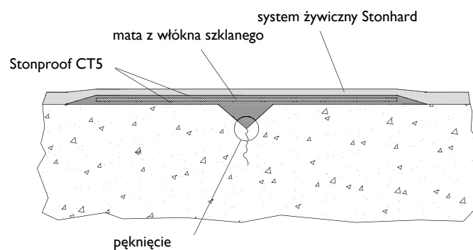
ZABEZPIECZENIE PĘKNIĘĆ Stonproof CT5 ze wzmocnieniem matą z włókna szklanego
