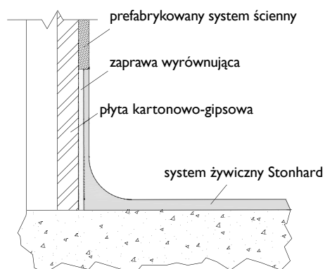
COKÓŁ SANITARNY Z PREFABRYKOWANYM SYSTEMEM ŚCIENNYM
